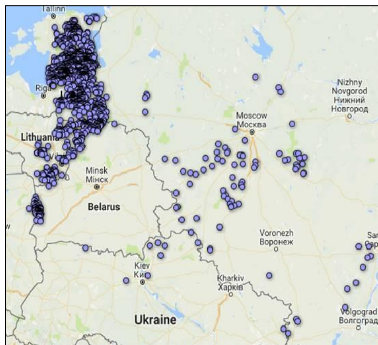
Obr. 3: Šírenie AMO v rokoch 2014-2016
