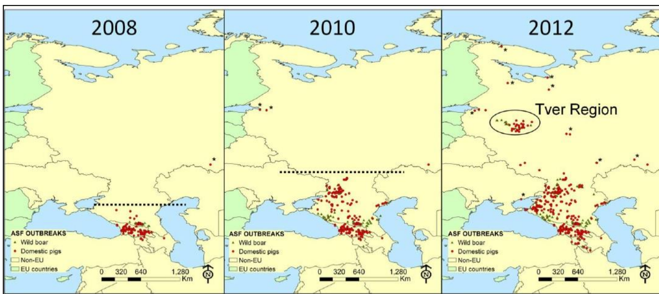
Obr. 1: Šírenie AMO v rokoch 2008-2012
