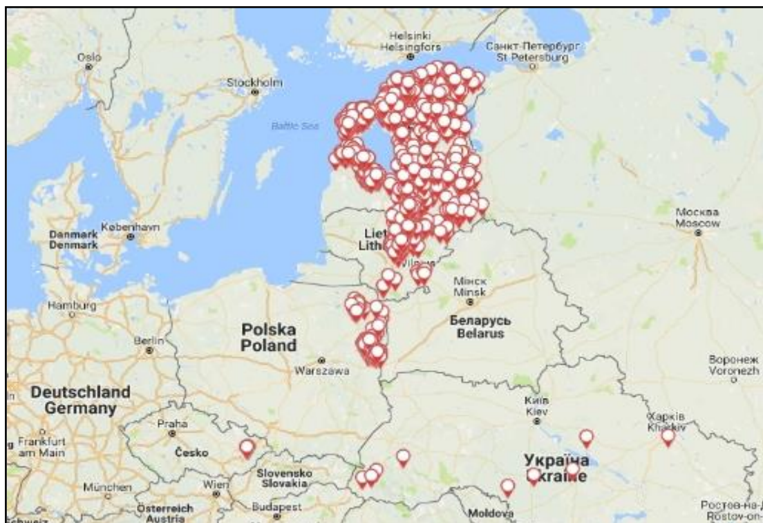
Obr. 5: Výskyt AMO v Európe k 17. 7. 2017
