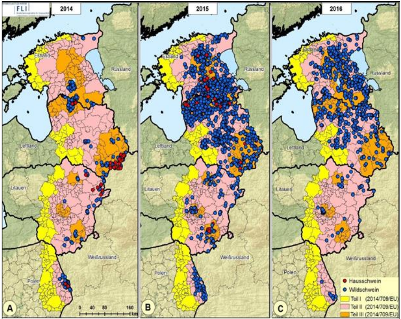
Obr. 5: Výskyt AMO v Európe k 17. 7. 2017
