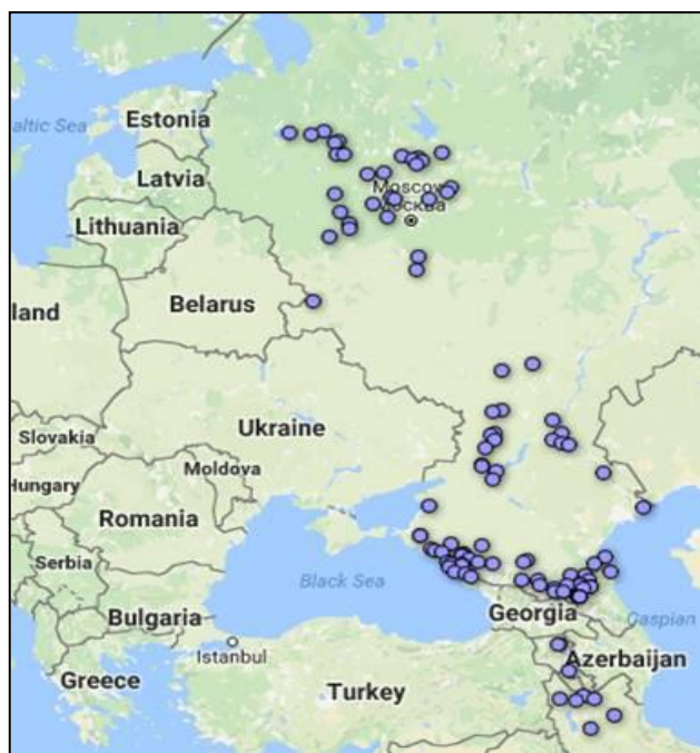
Obr. 2: Šírenie AMO v rokoch 2014-2016
